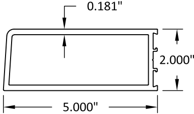
⑩④ HINGE STILE
