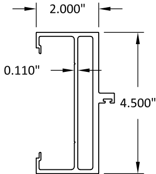
② DOOR JAMB O/P
